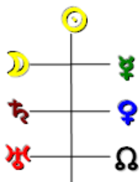
CONFIGURATION PLANÉTAIRE AXE SOLEIL
