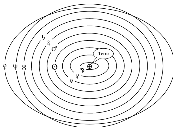
SYSTEME GEOCENTRIQUE.
